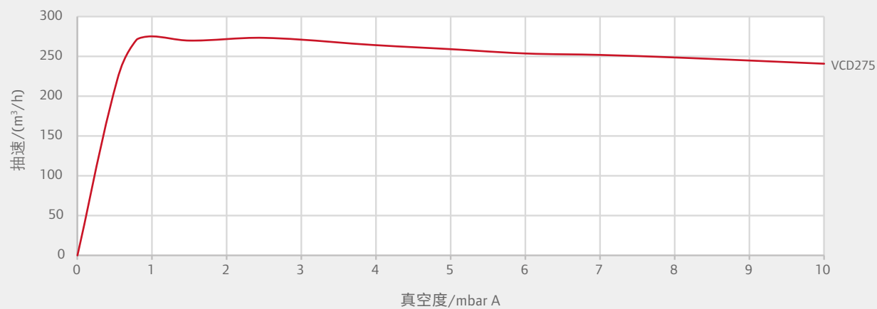
VCD275 性能曲线
