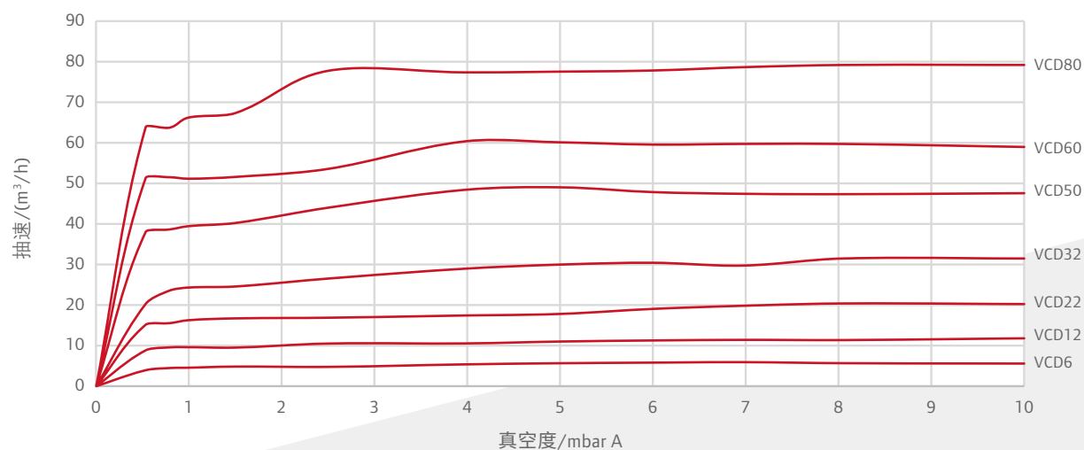
VCD6-80 性能曲线
